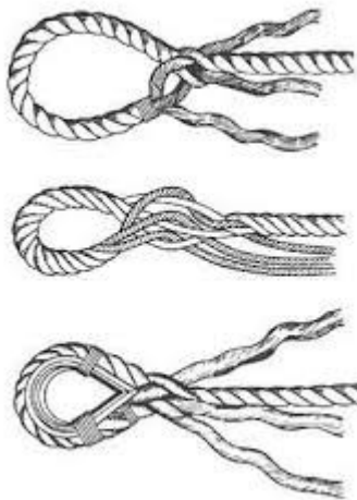
Augspleiß
